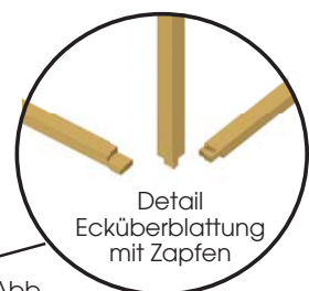
Abb. Konstruktion mit Fundamentrahmen
